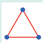
K_3
