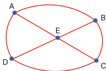
G_3
