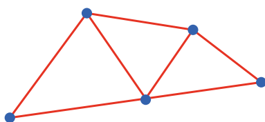
Grafo simples
