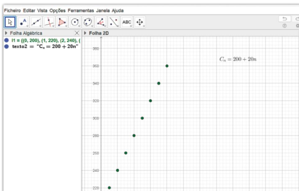
Representação da evolução do capital
