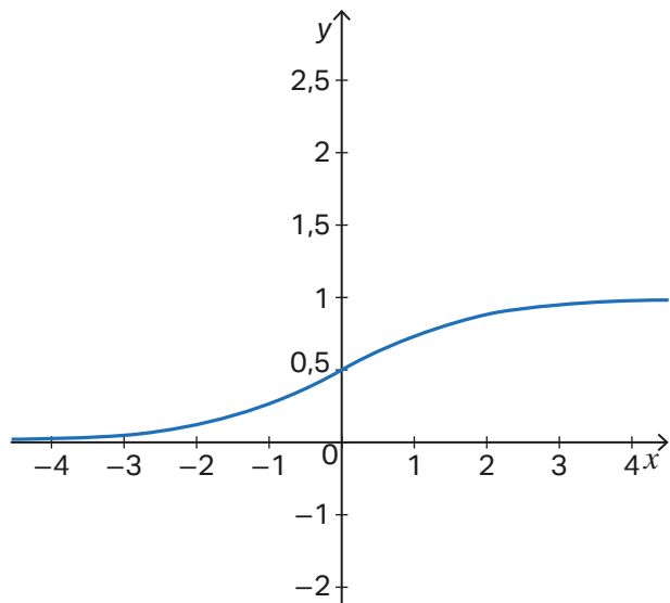
Função logística com todas as constantes iguais a 1.
