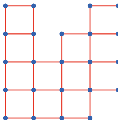
G_6
