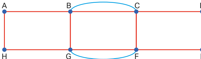
Exemplo 2 de eulerização do grafo
