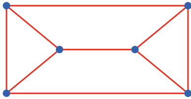
Grafo regular (todos os vértices têm grau 3)
