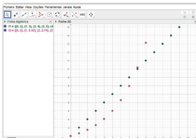
Um possível modelo discreto de Malthus.
