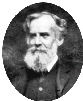
John Venn (1834-1923)
