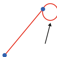
Multigrafo
