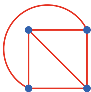
Grafo completo
