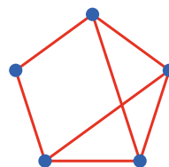
Grafo não completo
