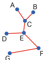
Árvore
