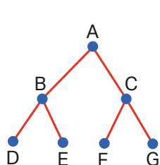
Árvore
