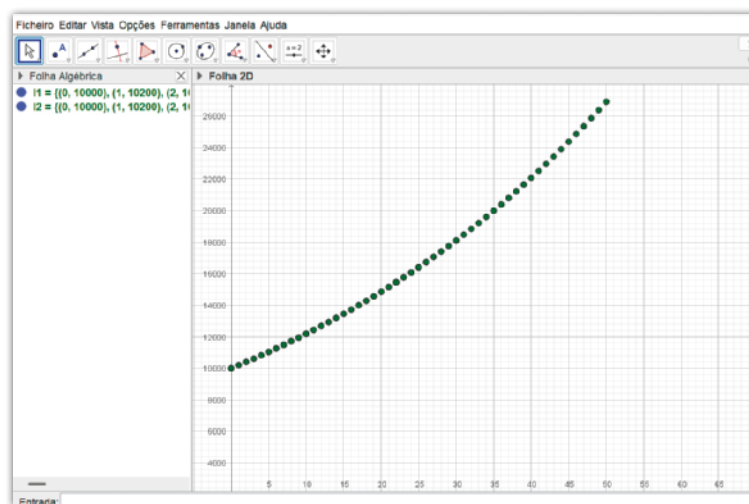
Os pontos do gráfico encontram-se sobre uma curva.
