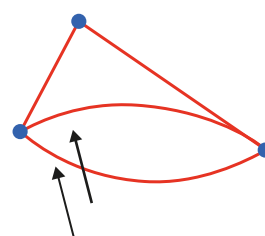
Multigrafo
