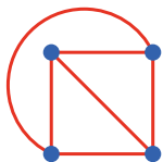
Grafo completo
