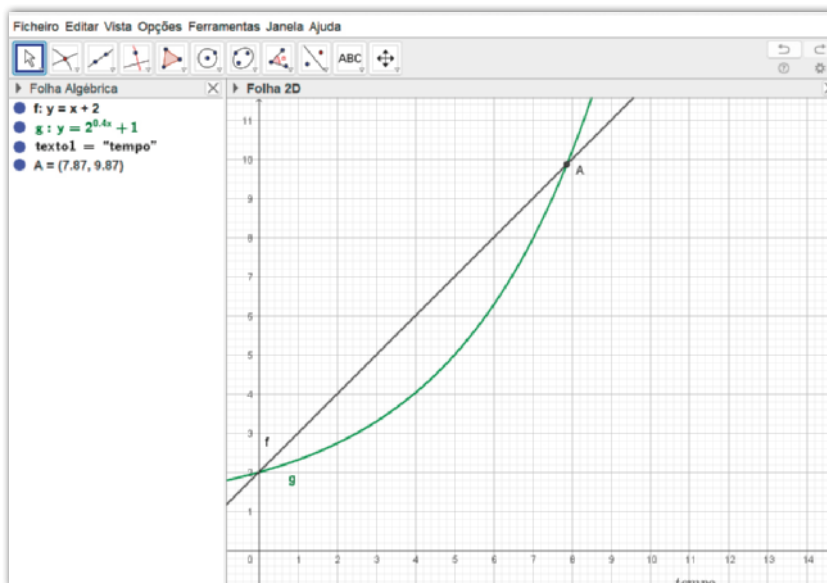
Um possível modelo contínuo de Malthus.
